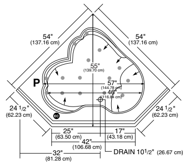
Système Tourbillon et Mass-air / Whirlpool & Mass-air System
