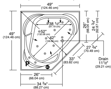
Système Tourbillon et Mass-air / Whirlpool & Mass-air System
